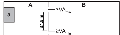
a Unitatea interioară A Încăperea în care este instalată unitatea interioară. B Încăperea învecinată cu încăperea A.
